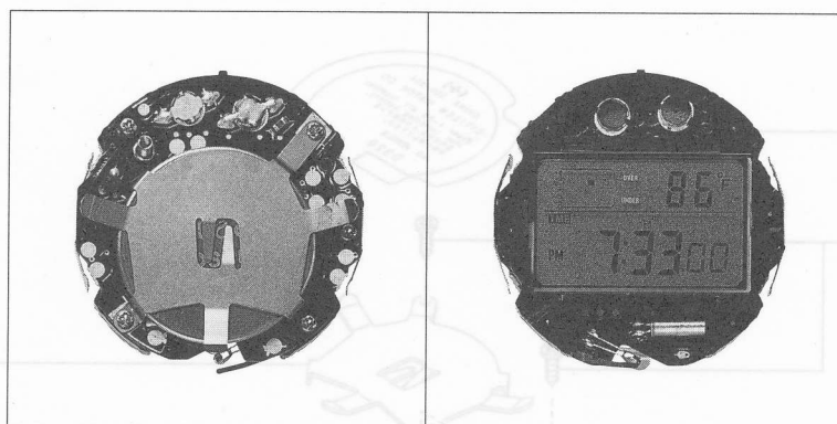
Caliber No. D320 キャリバー No. D320
